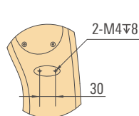
肘部孔位图 Elbow arm
