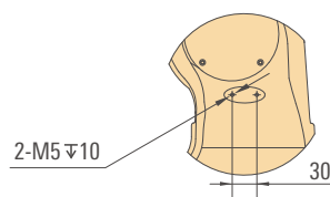
大臂孔位图 Lower arm
