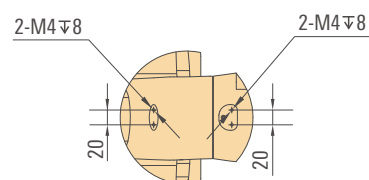
小臂孔位图 Upper arm
