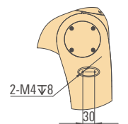
肘部孔位图 Elbow arm
