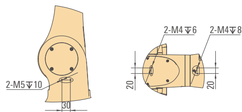
大臂孔位图 Lower arm
