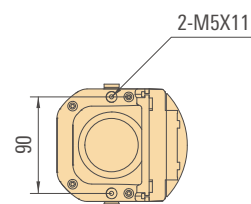
腕部孔位图 Wrist arm
