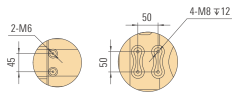
肘部孔位图 Elbow arm
