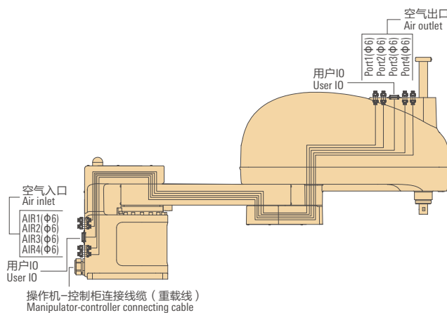
机体内配线 • 配管 Integrated dressing
