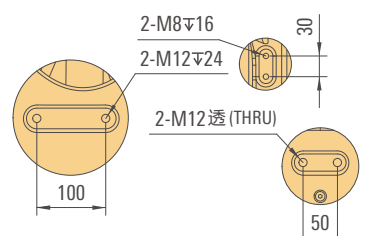
大臂孔位图 Lower arm
