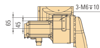
肘部孔位图 Elbow arm
