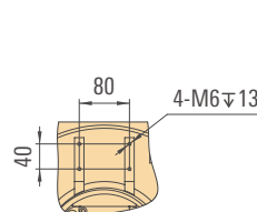
肩部孔位图 Shoulder arm
