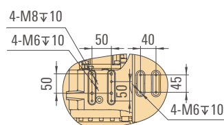
肘部孔位图 Elbow arm
