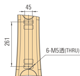
大臂孔位图 Lower arm
